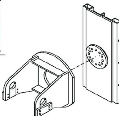
салазки с соединительным устройством стрелы
